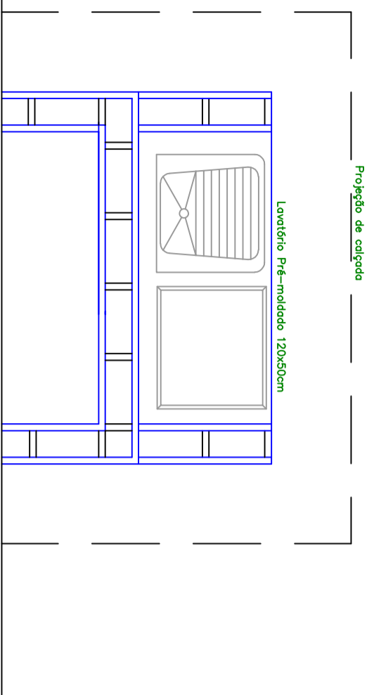
PLANTA BAIXA Esc: 1/20
