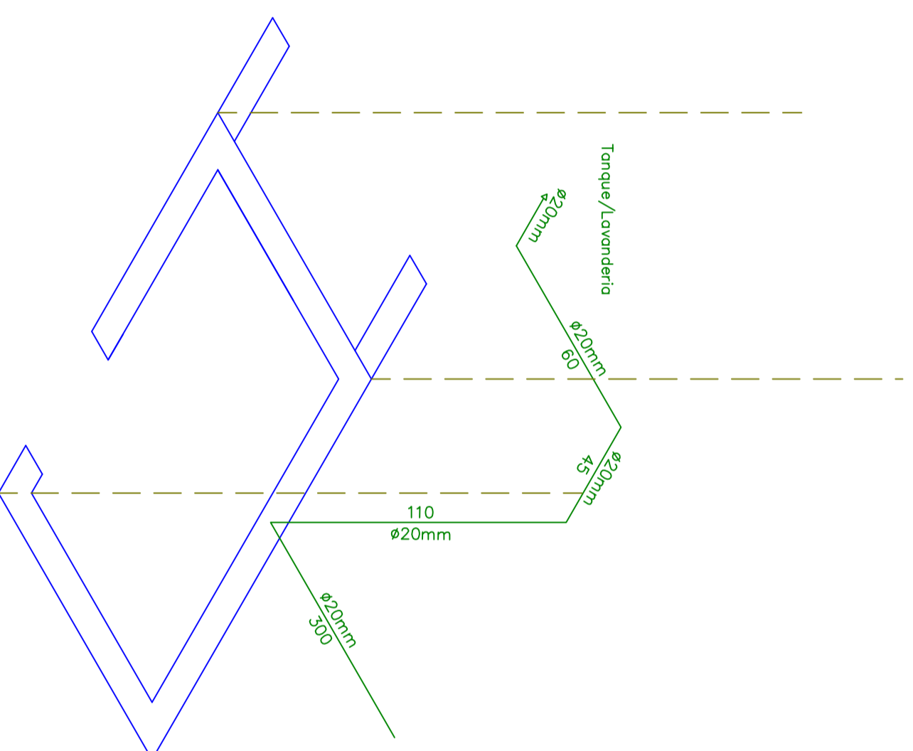
ISOMÉTRICA (TANQUE) Esc: 1/20
