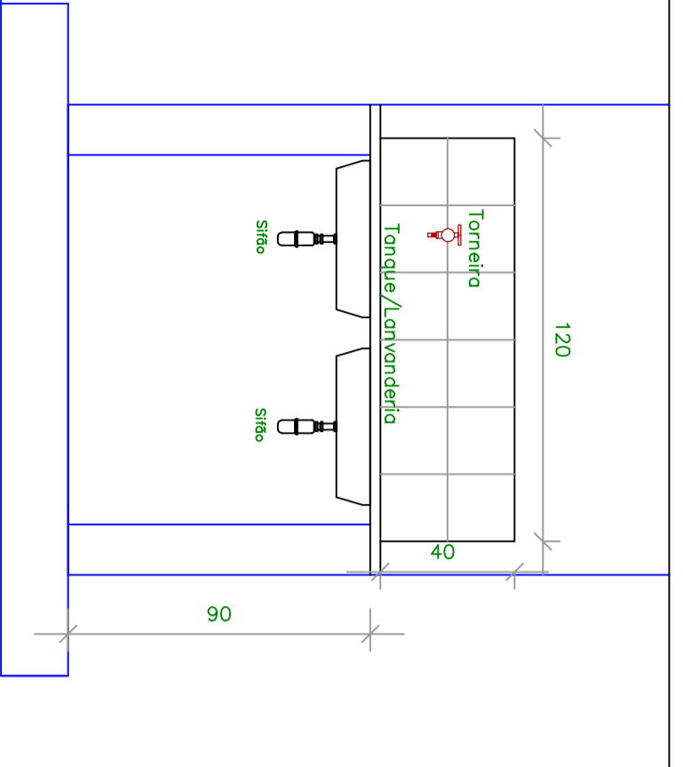
VISTA 01 Esc: 1/20
