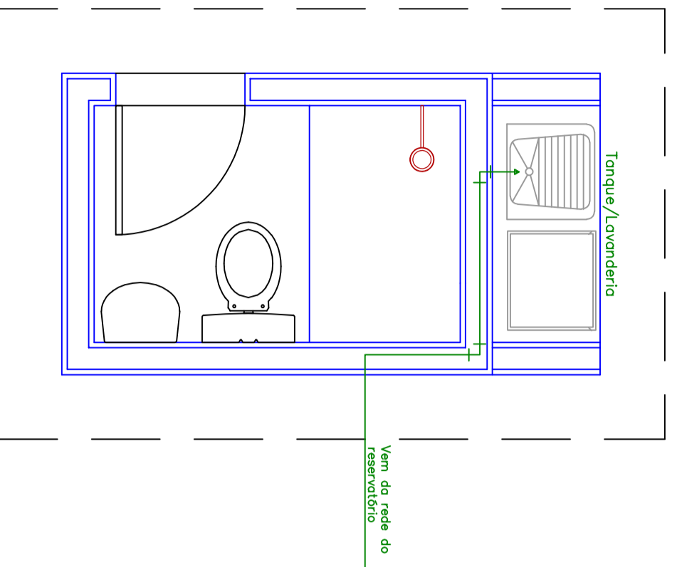
INSTALAÇÃO HIDRÁULICA (TANQUE) Esc: 1/25
