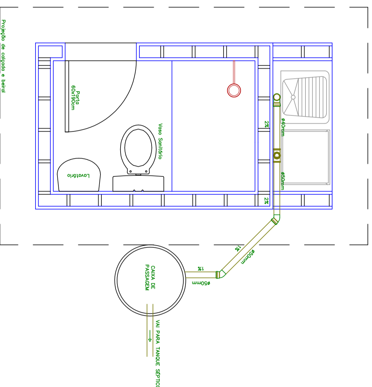
INSTALAÇÃO SANITÁRIA (TANQUE) Esc: 1/20
