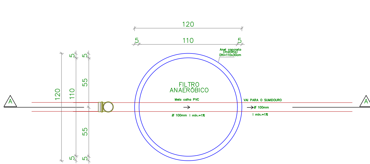
PLANTA BAIXA Esc: 1/20
