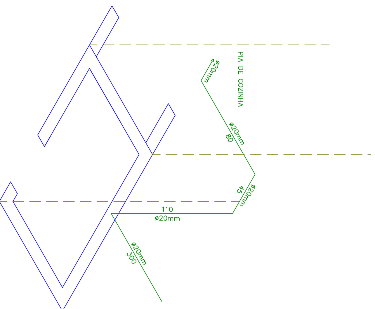
ISOMÉTRICA (PIA DE COZINHA) Esc: 1/20
