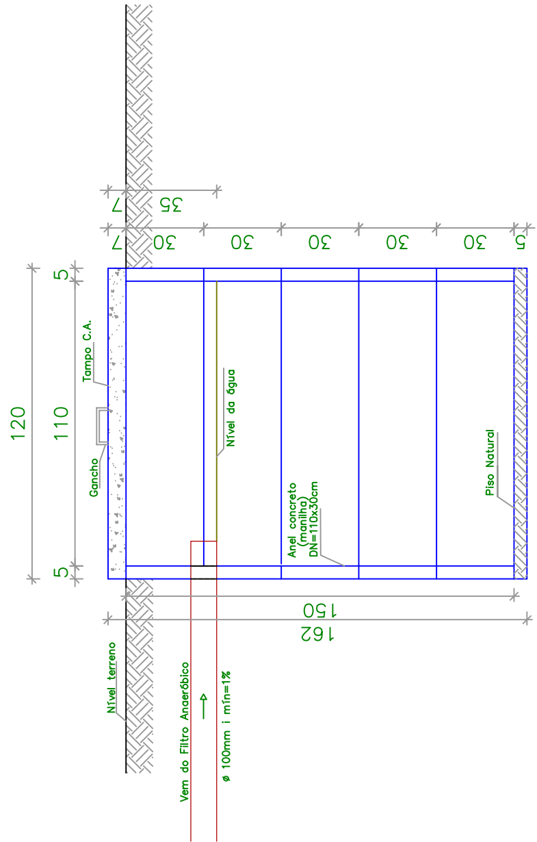
CORTE A--A
