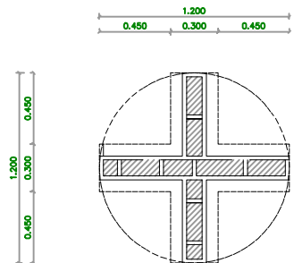
ALVENARIA RESERVATÓRIO
