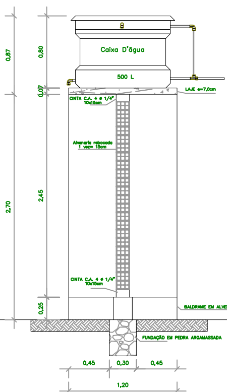
CORTE AA Esc: 1/30
