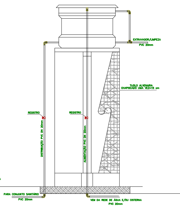
DETALHE DA LIGAÇÃO Esc: 1/30
