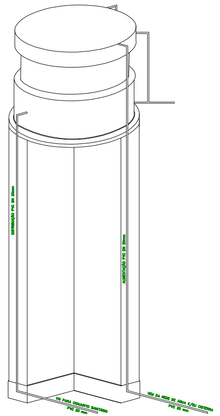
PERSPECTIVA Esc: 1/30
