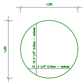
LAJE DE APOIO (1x) H=7cm RESERVATÓRIO
