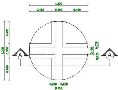
CINTAS (CORTE AA) RESERVATÓRIO
